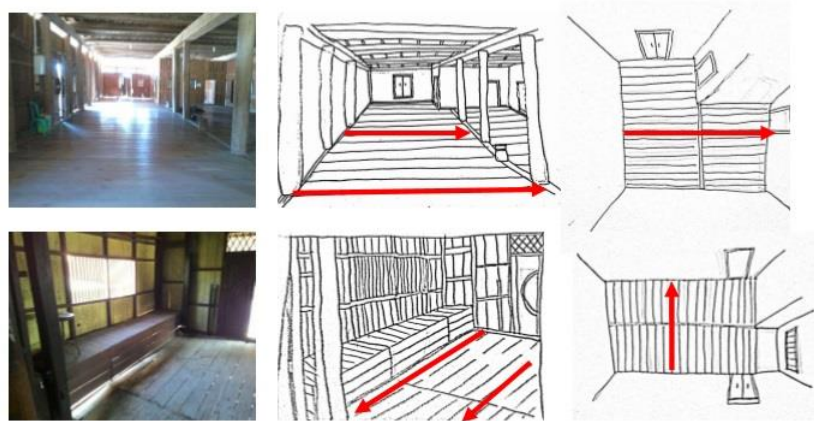
Gambar 5. Susunan Lantai
