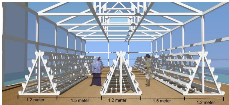
Gambar 10. Perspektif interior lab. Hidroponik
