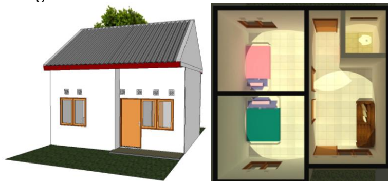
Gambar 2. Perspektif rekomendasi desain (kiri), denah ortogonal rekomendasi (kanan)
