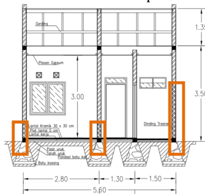
Gambar 4. Rencana dinding trasram pada potongan
