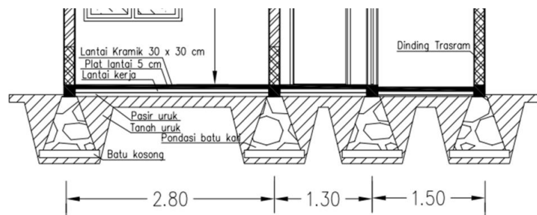
Gambar 3. Rencana rekomendasi plat lantai rumah tipe 36
