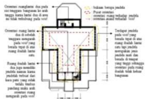
Gambar 21. Orientasi ruang lantai dua pada bangunan Gereja Kritis Indonesia Pregolan Bunder Surabaya tahun 1921.
