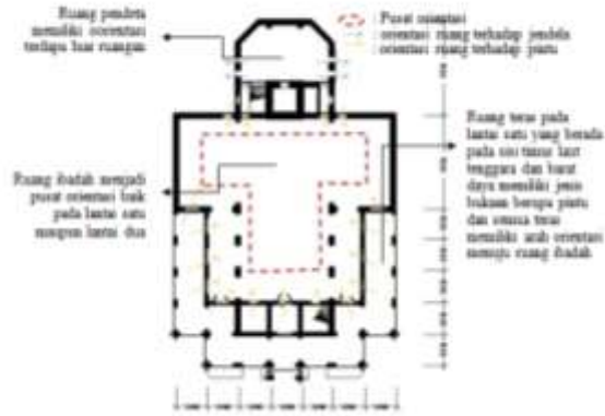
Gambar 20. Orientasi ruang lantai satu pada bangunan Gereja Kritis Indonesia Pregolan Bunder Surabaya tahun 1921.
