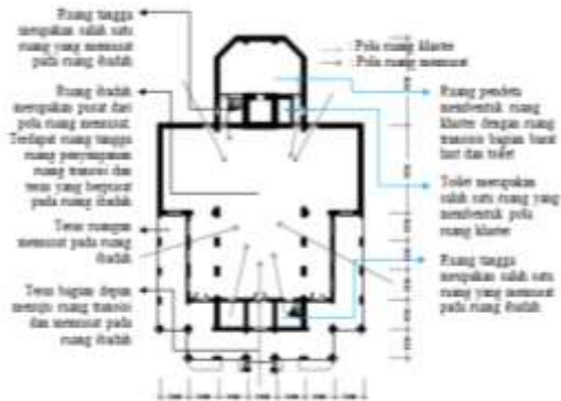
Gambar 12. Pola ruang lantai satu pada bangunan Gereja Kritten Indonesia Pregolan Bunder Surabaya tahun 1921
