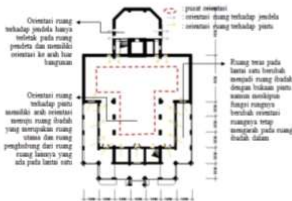
Gambar 22. Orientasi ruang lantai satu pada bangunan Gereja Kritis Indonesia Pregolan Bunder Surabaya tahun 2018.
