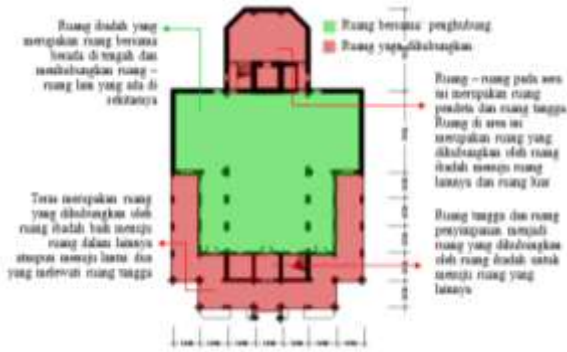
Gambar 7. Hubungan ruang yang dihubungkan oleh ruang bersama pada lantai satu Gereja Kriteen Indonesia Pregolan Bunder Surabaya tahun 1921
