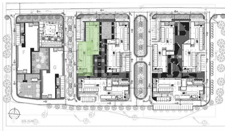
Gambar 1. Lokasi Blok H pada Siteplan Rusunawa Pesakih
