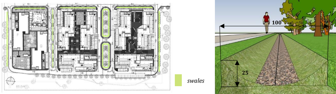
Gambar 3. Rekomendasi Keyplan dan Desain Swales
