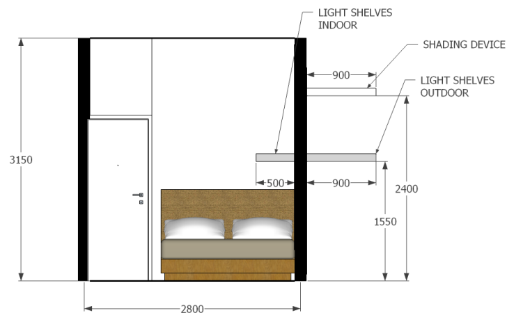
Gambar 8. Rekomendasi Desain Light Shelves pada Kamar Tidur
