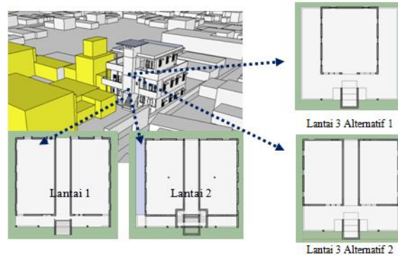
Gambar 13. Rekomendasi ruang kelas (Sumber: Hasil Analisis, 2014)
