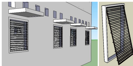
Gambar 14. Model Bukaan (Sumber: Hasil Analisis, 2014)
