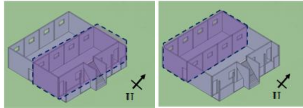
Gambar 7. Ruang Kelas 1 dan 2 (Sumber: Hasil Analisis, 2014)
