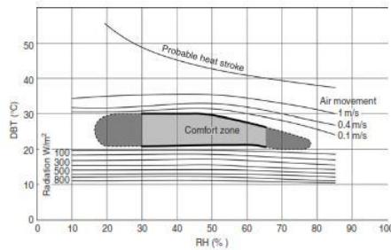
Gambar 3. Standar Efektif Temperatur
