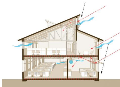
Gambar 4. Sistem Ventilasi silang pada bangunan
