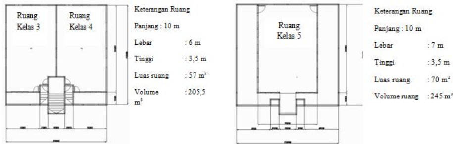
Gambar 10. Volume Ruang Kelas 3, 4 dan 5 (Sumber: Hasil Analisis, 2014)
