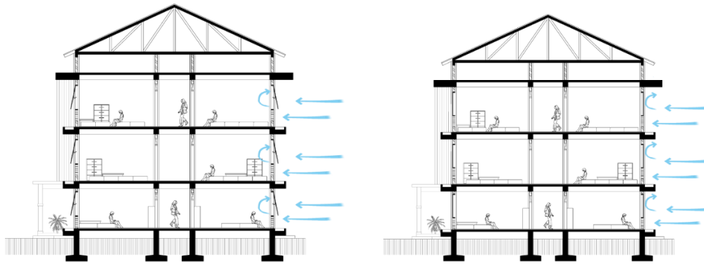
Gambar 2. Gambar potongan bangunan rusunawa terhadap aliran angin pada saat jendela dibuka dan ditutup
