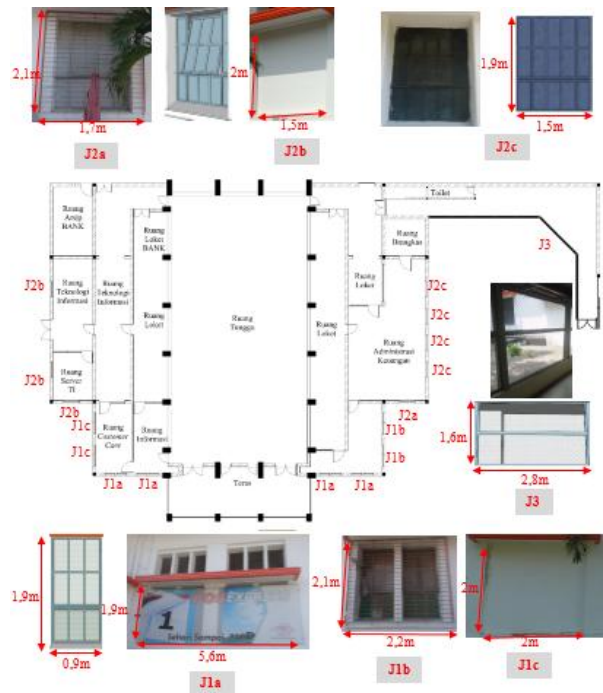
Gambar 10. Jendela
