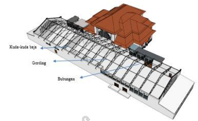
Gambar 15. Konstruksi atap
