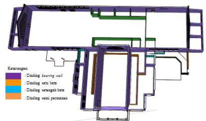
Gambar 16. Konstruksi dinding
