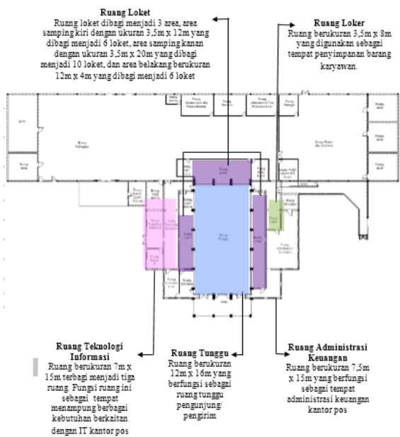
Gambar 4. Fungsi ruang
