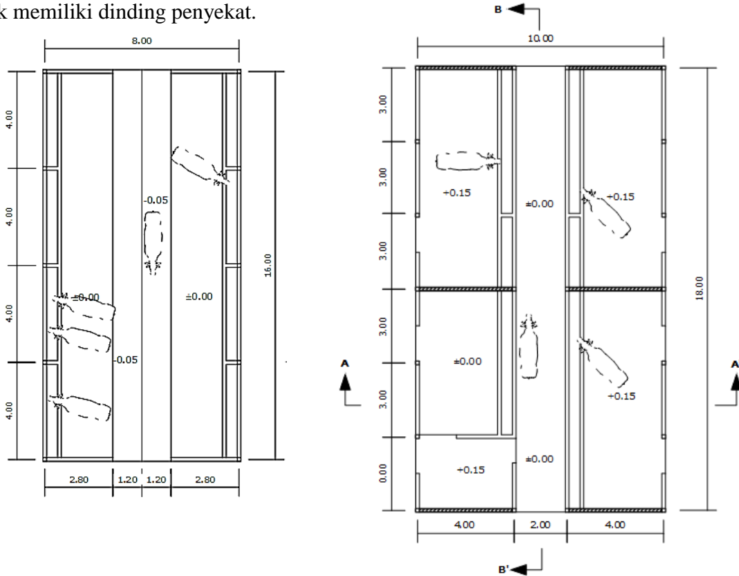
Gambar 2 Denah kandang terbuka dan semi terbuka
