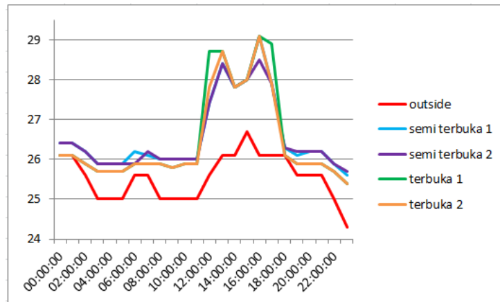
Grafik 3 Perbandingan suhu hasil simulasi
