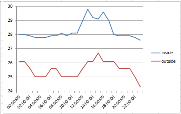
Grafik 2 Validasi suhu kandang semi terbuka
