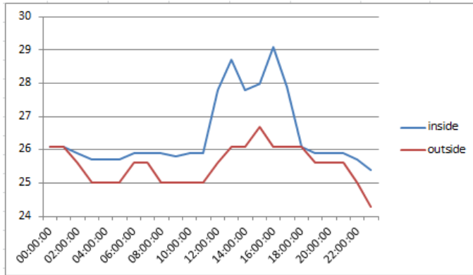
Grafik 1 Validasi suhu kandang terbuka
