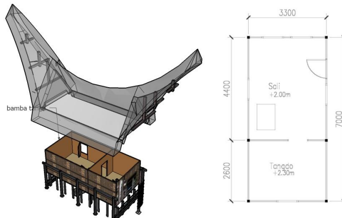
Gambar 5. Tongkonan Batu A'Riri
