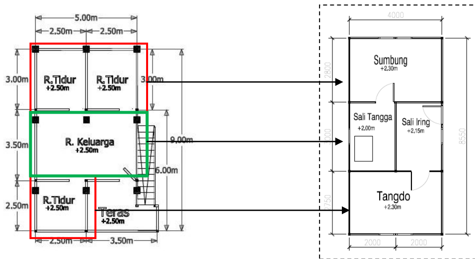
Gambar 6. Banua Barung-barung I awal dan Tongkonan Layuk
