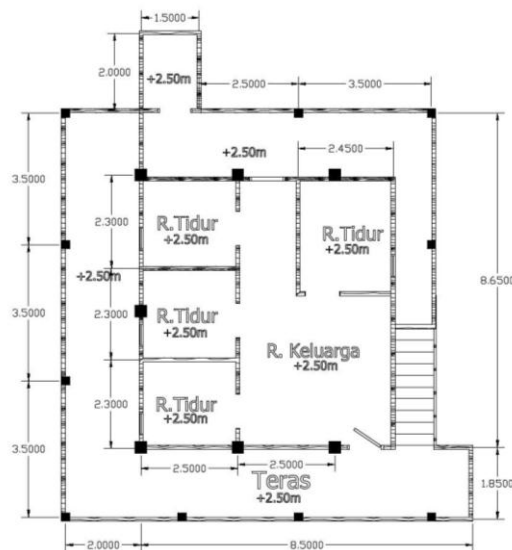
Gambar 7. Banua Barung-barung setelah penambahan
