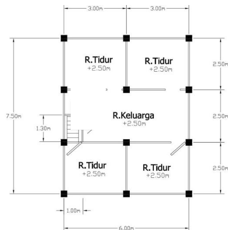
Gambar 9. Banua Barung-barung II setelah penambahan
