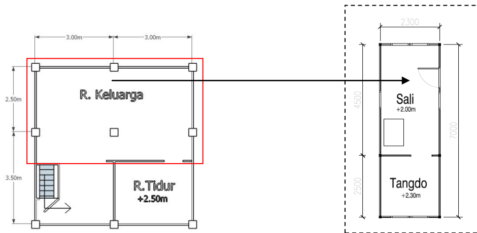
Gambar 8. Banua Barung-barung II awal dan Tongknan Batu A'Riri
