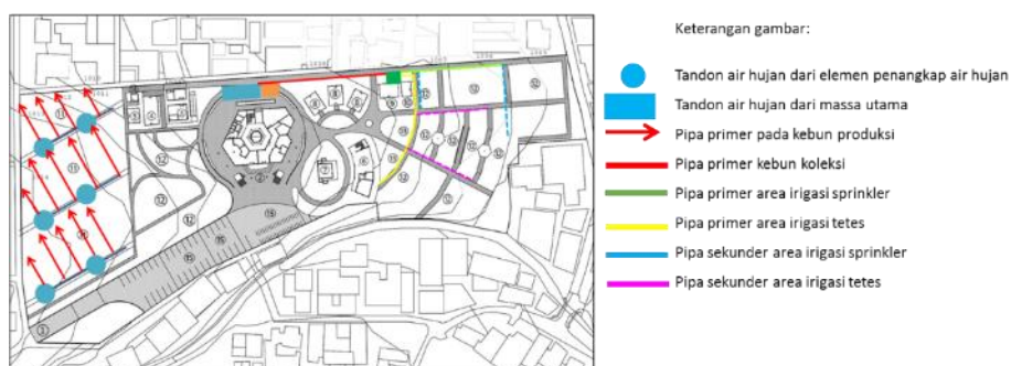
Gambar 7. Sistem Distribusi Air Hujan untuk Kegiatan Penyiraman (Sumber: Hasil analisis, 2015)
