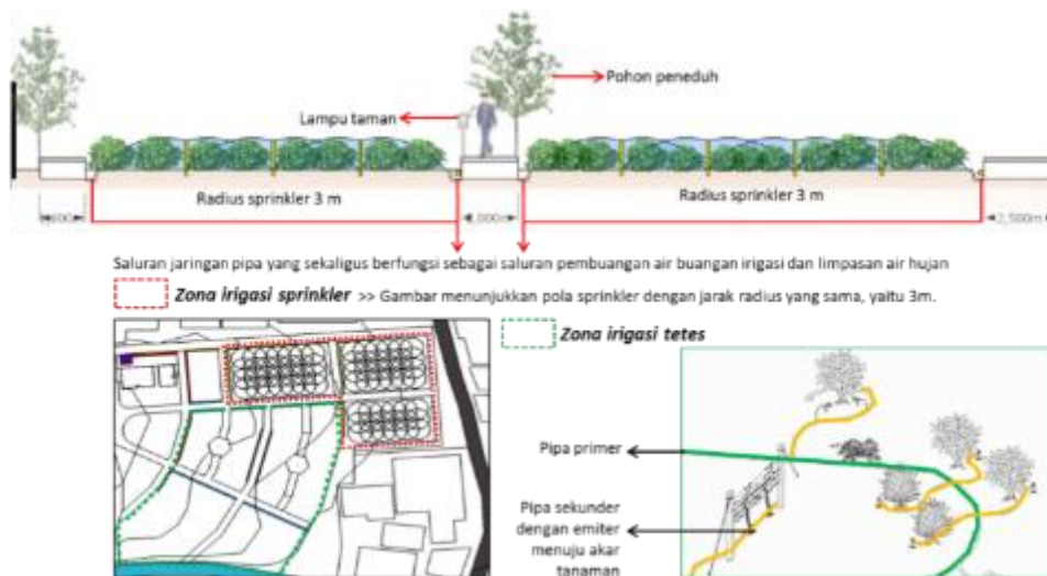
Gambar 8. Sistem Penyiraman pada Kebun Koleksi (Sumber: Hasil analisis, 2015)
