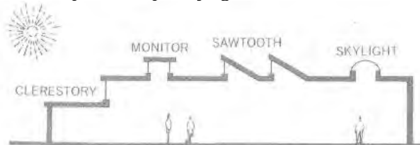
Gambar 2. Jenis-jenis Toplighting
