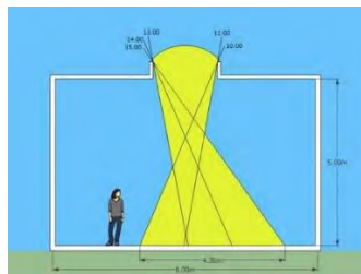
Gambar 10. Simulasi Masuknya Cahaya melalui Top Lighting Skylight pada Bulan Desember
