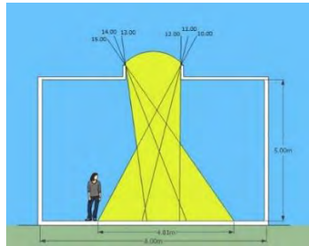
Gambar 8. Simulasi Masuknya Cahaya melalui Top Lighting Skylight pada Bulan Maret
