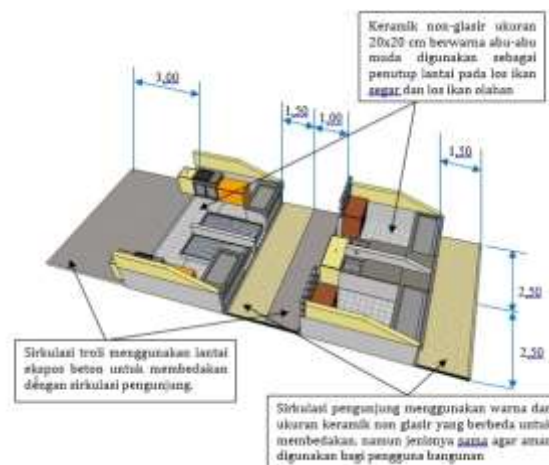
Gambar 6. Konsep Penerapan Material Lantai pada Pasar Ikan (Sumber: Hasil analisis, 2014)
