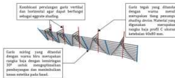
Gambar 2. Konsep Pembayangan pada Bangunan (Sumber: Hasil analisis, 2014)
