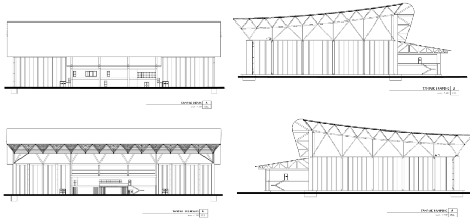
Gambar 3. Tampak Bangunan
